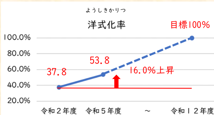
洋式便器
